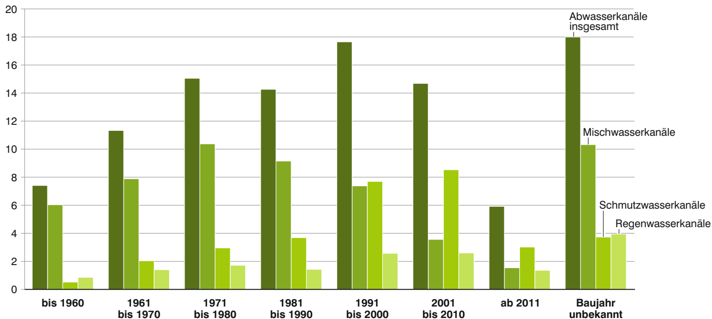
Abb. 16 Länge des Kanalnetzes in Bayern 2016 nach Art und Baujahr in Tausend km
